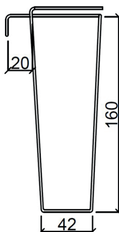
Staande strek Type SfLH/I-160
